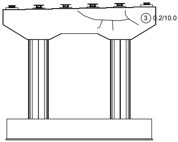
전면
